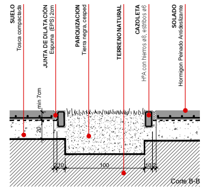
Corte B-B
